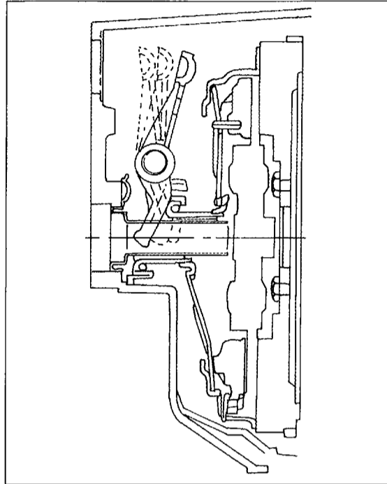
Bild 198 Schnitt durch die Kupplung, wenn das Ausrücklager gezogen wird (mit MG5TU-Getriebe).
