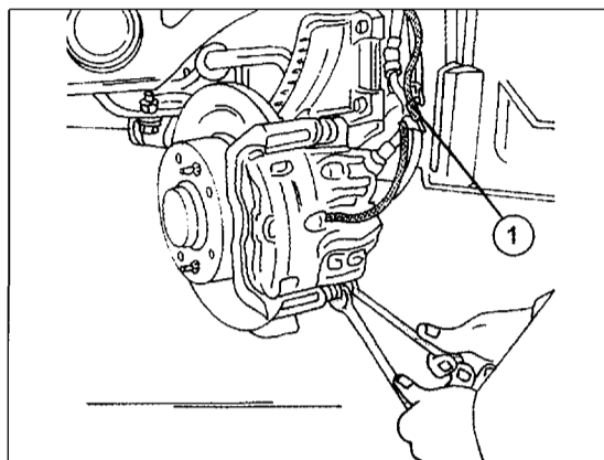
Bild 290 Das Kabel der Verschleißanzeige für die Bremsklötze (1) muss an der gezeigten Stelle getrennt werden.
