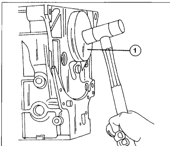
Bild 107 Einschlagen des hinteren Öldichtringes. 1 Platte
