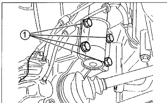
Bild 223 Die vier mit den Pfeilen gezeigten Schrauben (1) halten das Federbein am Achsschenkel, Querlenker, usw. verbleiben beim Ausbau des Federbeins an der Radaufhängung.
