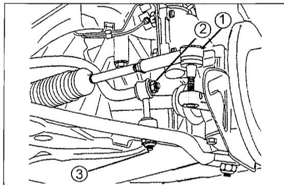
Bild 269 Anschlussweise der Koppelstange des Kurvenstabilisators und der Spurstange.
