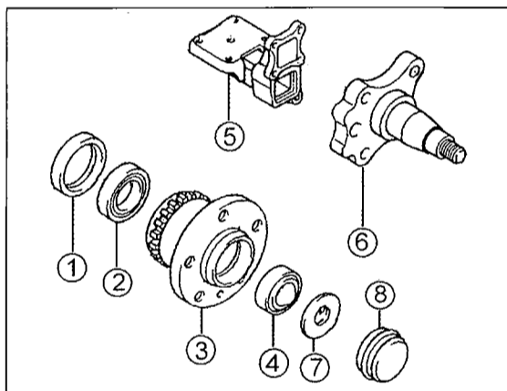
Bild 251 Radnabe und Radlager (ohne Radlagermutter). 1 Öldichtring 2 Inneres Radlager 3 Radnabe mit Zahnkranz (ABS) 4 Äußeres Radlager 5 Hinterachskörper 6 Achsstumpf 7 Unterscheibe 8 Nabenfettkappe
