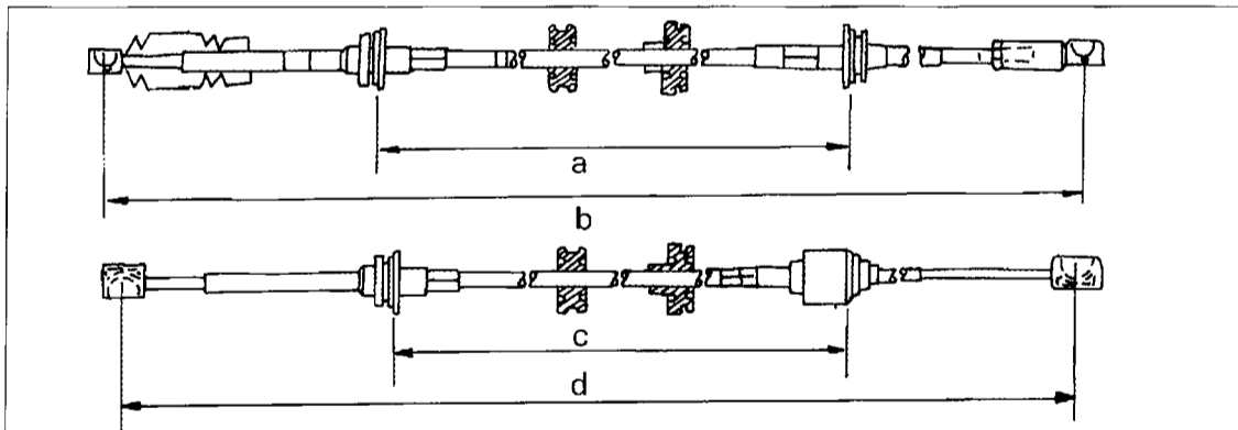
Bild 211 Die Einbaumaße der beiden Schaltseile. Oben das Gangwählseil, unten das Gangschaltseil. Maßangaben „a“ bis „d“ sind dem Text zu entnehmen. Die Maße sind bei den verschiedenen Getrieben unterschiedlich.
