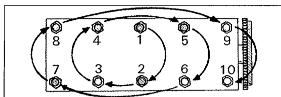
Bild 66 Reihenfolge zum Festziehen der Zylinderkopfschrauben eines 2.0-Liter-Motors. Die Schrauben in entgegengesetzter Reihenfolge lockern.
