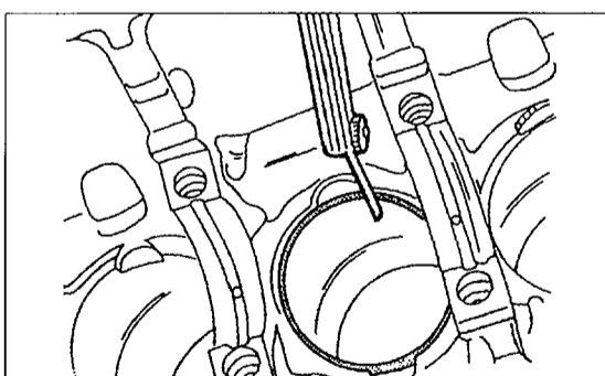
Bild 99 Ausmessen des Stoßspiels der Kolbenringe. Das Spiel kann gemessen, aber nicht verändert werden.
