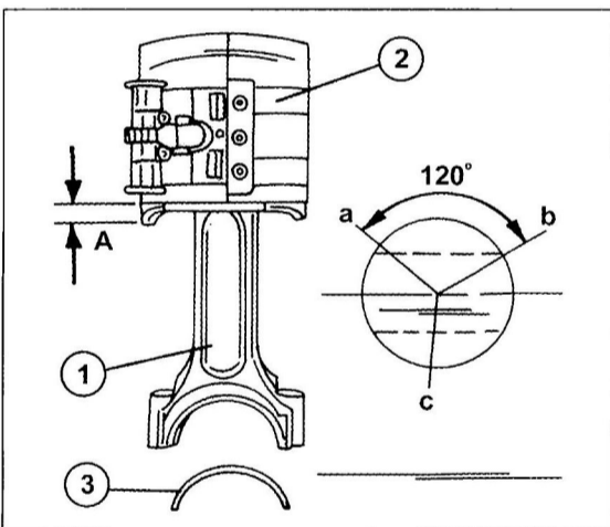
Bild 102 Zum Einbau der Kolben- ringe. Stöße „a“ bis „c“ in gezeigter Weise anordnen. Der Kolben muss an Stelle „A“ aus dem Spannband herausstehen. 1 Pleuellstangen/ Kolbeneinheit 2 Kolbenringspannband 3 Pleuellagerschale
