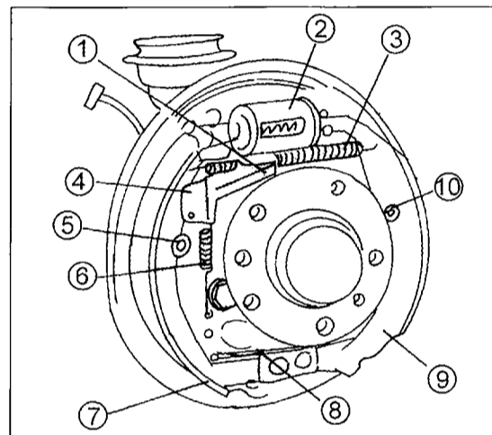
Bild 300 Ansicht einer Hinterradbremse. 1 Druckstange des Verstellmechanismus 2 Radbremszylinder 3 Obere Backenrückzugfeder 4 Verstellhebel 5 Backenankerstift 6 Hebelrückzugfeder 7 Bremsbacken 8 Untere Backenrückzugfeder 9 Bremsbacken 10 Backenankerstift
