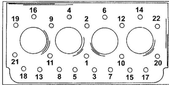
Bild 40 Reihenfolge zum Anziehen der Zylinderkopfschrauben. Die Schrauben werden in umgekehrter Reihenfolge gelockert.
