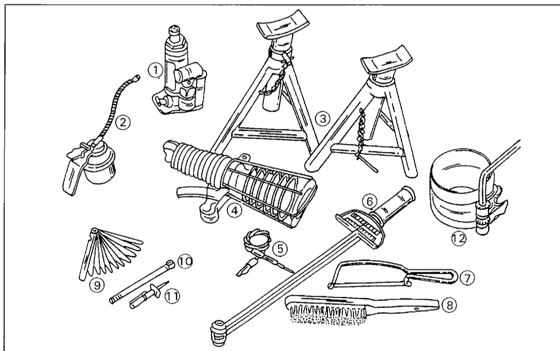
Bild 11 Vorgeschlagene Werkzeuge und Hilfswerkzeuge zur Pflege und Reparatur Ihres Fahrzeuges. 1 Hydraulischer Heber 2 Ölkanne 3 Unterstellböcke 4 Elektrische Handlampe 5 Prüflampe (12 Volt) 6 Drehmomentschlüssel 7 Minisäge 8 Drahtbürste 9 Blattfühlerlehren 10 Reifendruckprüfer 11 Reifenprofilmesser 12 Kolbenringspannband
