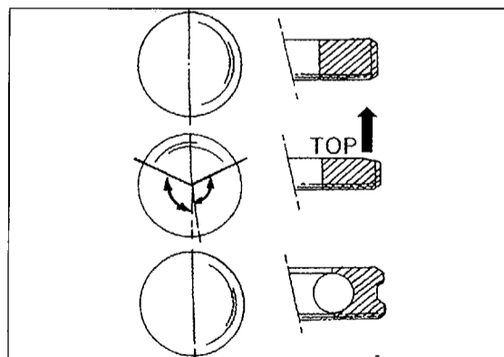
Bild 95 Anordnung der Kolbenringe. Zu beachten ist die Einbauweise des zweiten Ringes.
