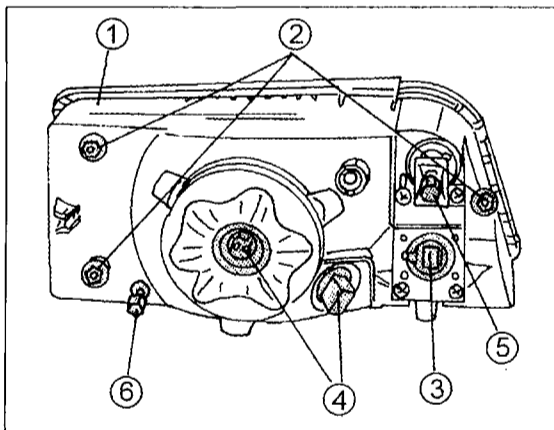
Bild 321 Ansicht der Rückseite eines Scheinwerfers. 1 Scheinwerfereinsatz 2 Befestigungsschrauben, Scheinwerfer 3 Stecker, Leuchtweitenverstellung 4 Stecker, Scheinwerfer und Standlicht 5 Höheneinstellschraube, Scheinwerfer 6 Seiteneinstellschraube, Scheinwerfer
