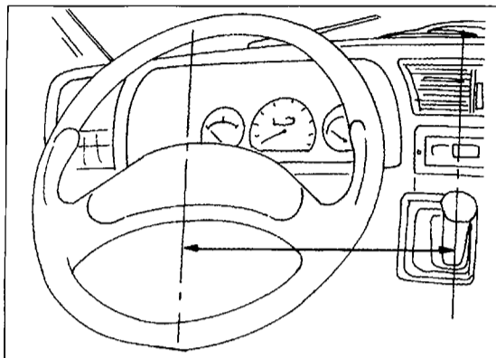
Bild 210 Das Maß wird zwischen den Pfeilen ausgemessen. Beträgt es 304 mm, stimmt die Einstellung.
