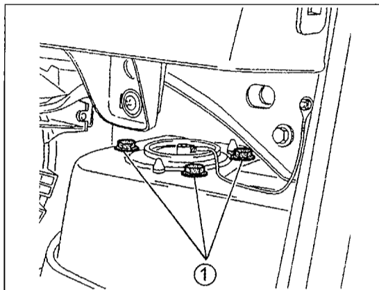
Bild 222 Die drei Schrauben (1) halten die Federbeineinheit (2) in der Innenseite des Fahrzeuges.
