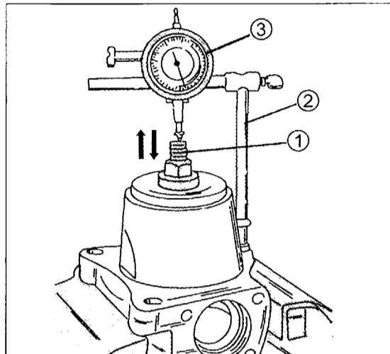
Bild 232 Kontrolle des Axialspiels der Radlager. Die mit einem Halter (2) angebrachte Messuhr (3) so ansetzen, dass der Messuhrstift auf die eingesezte Schraube (1) aufsitst. Durch Hin- und Herbewegen der Schraube (Pfeile) wird das Spiel an der Messuhr angezeigt.
