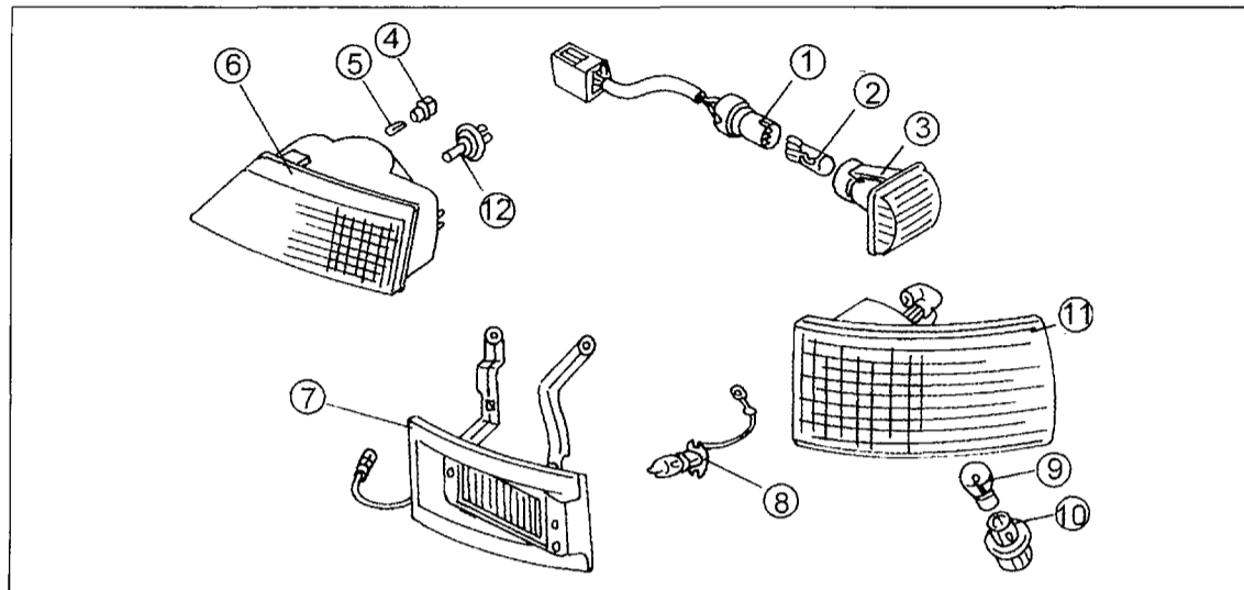
Bild 319 Die verschiedenen Leuchten an der Vorderseite des Fahrzeuges. 1 Kabelstecker und Kabel für Seitenblinkleuchte 2 Glühbirne, Seitenblinkleuchte 3 Seitenblinkleuchte 4 Birnenfassung, Standlicht 5 Glühbirne, Standlicht 6 Scheinwerfer 7 Nebelleuchte 8 Glühbirne, Nebelleuchte 9 Glühbirne, Blinkleuchte 10 Glühbirnenfassung, Blinkleuchte 11 Blinkleuchte 12 Glühbirne, Scheinwerfer
