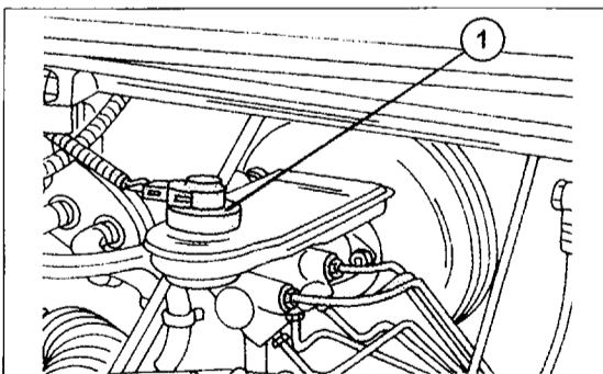
Bild 331 Durch Druck auf den gezeigten Verschlussdeckel kann man die Arbeitsweise der Warnleuchte für die Bremsflüssigkeit kontrollieren.
