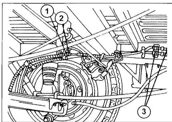
Bild 247 Ansicht der Unterseite des Fahrzeuges bei ein- gebauter ABS-Anlage. 1 Federspanne zur Schlauchhalterung 2 Bremschlauch- anschluss 3 Kabelstecker für Raddrehzahlsensoren
